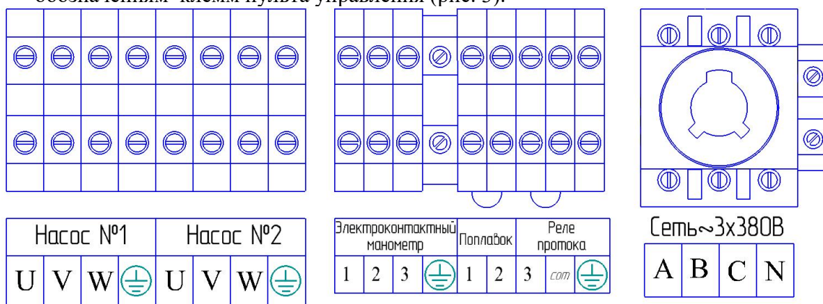
Рис. 3 Обозначение клемм пульта управления.
