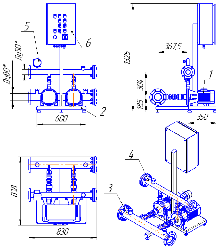
Рис.1 Внешний вид станции.
